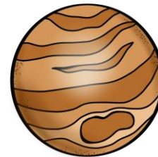
Iúpatar
