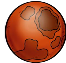
Mars
