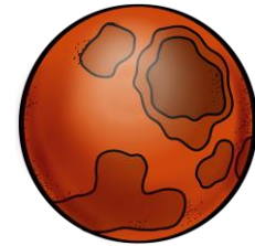
Mars
